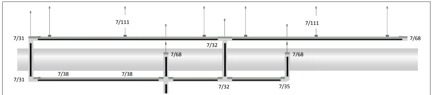
Colocación y fijación en superficie por coliso de guía o con grapas auxiliares 7/38 y en suspensión con tensores metálicos 7/111.
